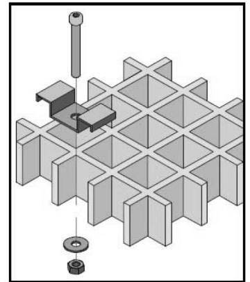
M-Clip
